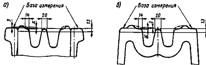
Рис. 3.19. Измерение вертикального износа x усювиков сборной (а) и цельнолитой (б) острых крестовин
