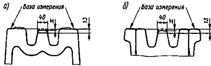
Рис. 3.17. Измерение вертикального износа x сердечника цельнолитой (а) и сборной (б) крестовины
