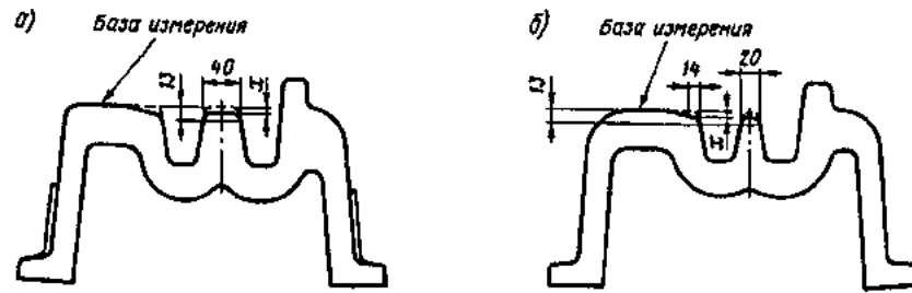
Рис. 3.18. Измерение вертикального износа x сердечника (а) и усювиков (б) цельнолитой тупой крестовины
