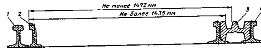
Рис. 3.23. Схема измерения расстояний между рабочими гранями контроельса и усювика и рабочими гранями контроельса и сердечника крестовины: 1 — путевоый рельс; 2 — контроельс; 3 — сердечник; 4 — усювик
