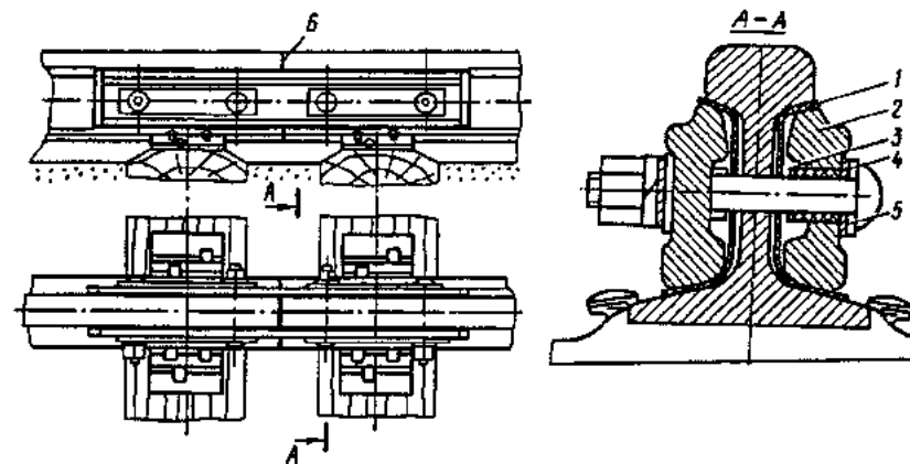
Рис. 3.39. Изолирующий стык с двухголовыми металлическими накладками для пути с деревянными шпалами: 1 — боковая прокладка; 2 — накладка; 3 — втулка; 4 — изолирующая планка под болт; 5 — столпорная планка; 6 — торцовая прокладка
