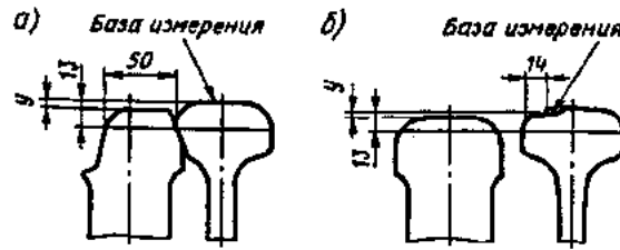
Рис. 3.25. Измерение понижения остряка относительно рамного рельса у при равномерном (а) и неравномерном (б) вертикальном износе рамного рельса
