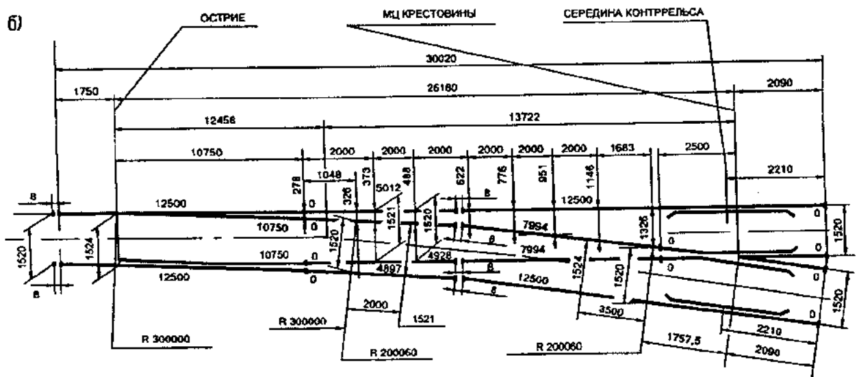
Рис. 5.13. Эюра укладки (а) и схема разбивки (б) стрелочного перевода типа Р65 марки 1/9. Проекты 2244 и 2772
