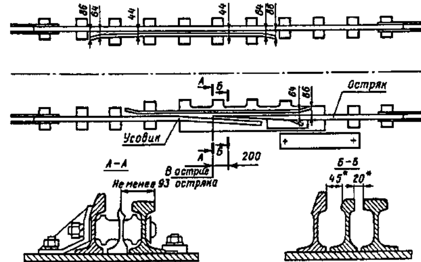
Рис. 3.29. Башмакосбрасыватели типов Р50, Р65 колен 1520 мм: * — на расстоянии 200 мм от остряка и до конца усовика
