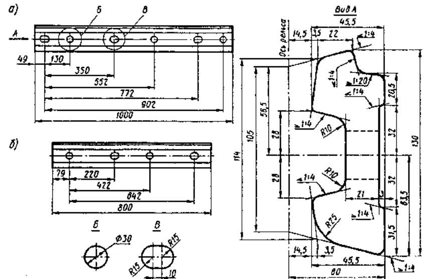
Рис. П.2.1. Накладка двухголовая к рельсам типов P65 и P75: а — шестидырная; б — четырёхдырная
