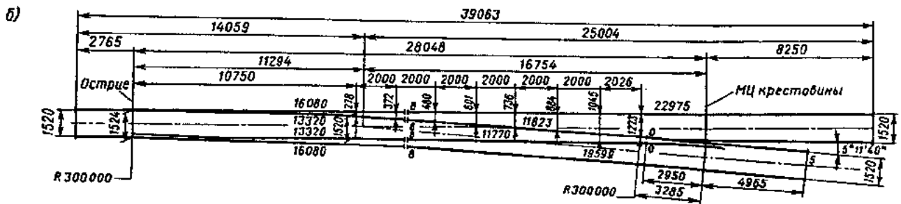
Рис. 5.3. Эпюры укладки (правосторонняя и левосторонняя) (а) и схема разбивки (б) стрелочного перевода типа Р65 марки 1/11 на железобетонных брусках для скоростного движения. Проект 2726
