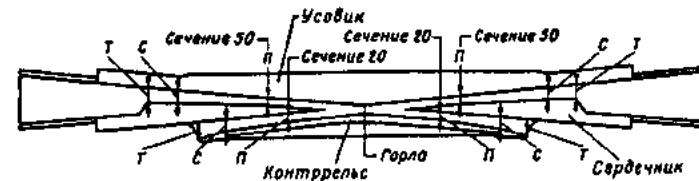
Рис. 3.14. Места контрольных измерений ширины желобов в тупых крестовинах (измерения проводятся в местах видимых передофов контррельса и нерабочей грани сердечника)
