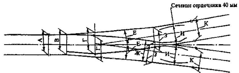
Рис. 3.10. Места контрольных измерений ширины колес на симметричных стрелочных переводах
