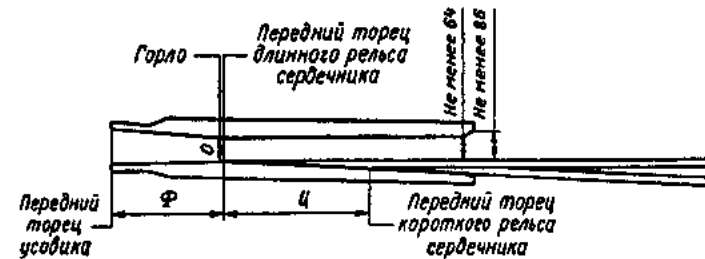
Рис. 3.13. Места контрольных измерений ширины желобов и расстояний от переднего торца усювика до переднего торца длинного рельса сердечника (Ф) и между торцами длинного и короткого рельса сердечника (Ц) на крестовинах с подвижным сердечником
