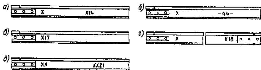
Рис. 3.6. Маркировка дефектных (а — г) и острodefектных (д) рельсов в зависимости от расположения дефекта: а — вне стыка; б — по всей длине рельса; в — на левом конце рельса; г — на правом конце рельса; д — вне стыка
