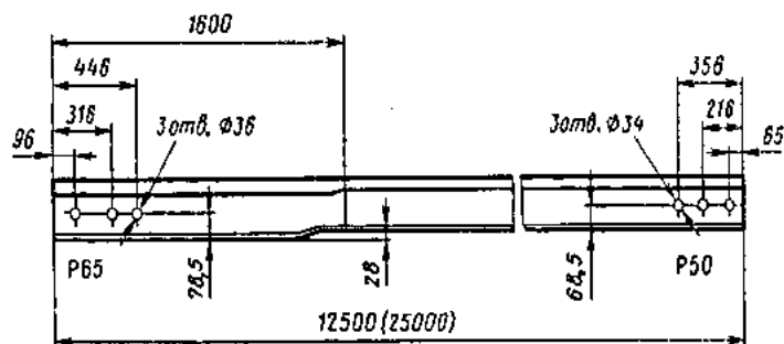
Рис. 3.3. Переходной рельс типа Р65/Р50
