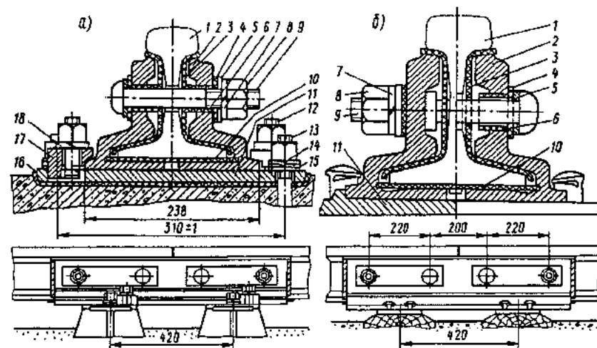
Рис. 3.38. Изолирующий стык с объемлющими металлическими накладками: а — при железобетонных шпалах и скреплении КБ; б — при деревянных шпалах с костыльным скреплением: 1 — рельс; 2 — накладка; 3 — прокладка боковая; 4 — подштыленовая планка под болты; 5 — металлическая столпорная планка; 6 — втулка; 7 — пружинная шайба; 8 — гайка; 9 — стыковой болт; 10 — изолирующая прокладка под рельс; 11 — подкладка; 12 — клеммный болт; 13 — закладной болт; 14 — пружинная шайба; 15 — плоская шайба; 16 — прокладка под подкладку; 17 — клемма; 18 — шайба
