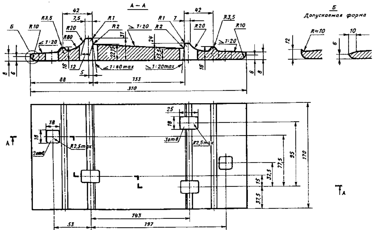
Рис. П.2.8. Подкладка Д50 костьельного скрепления к рельсам типа Р50
