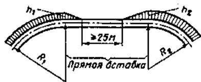
Рис. 2.2. Схема отводов возвышения наружной рельсовой нити при сопряжении смежных кривых одного направления при достаточной длине прямой вставки между ними
