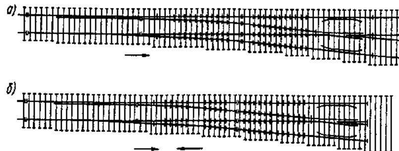
Рис. 3.27. Схема закрепления от угона стрелочного перевода марок 1/11 и 1/9 пружинными противоугонами при одностороннем (а) и двухстороннем (б) движении поездов
