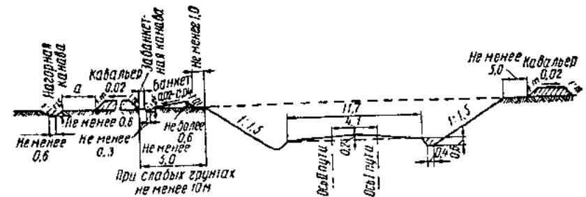
Рис. П.6.4. Выемка глубиной до 12 м с шириной основной площадки 11,7 м при поперечном уклоне местности не круче 1:3
