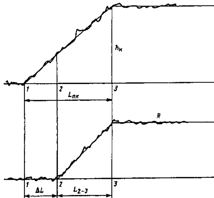
Рис. 2.6. Несовпадение ( \Delta L ) начала возвышения наружного рельса с началом кривизны ( L_{2-3} < L_{kk} ) на ленте путеизмерителя
