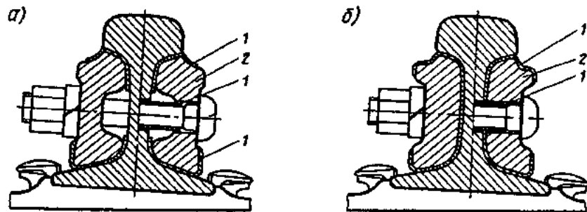
Рис. 3.40. Клеebolтовой изолирующий стык при костыльном скреплении: а — с двухголовыми металлическими накладками; б — со специальными (полнопрофильными) накладками; 1 — изолирующий слой; 2 — накладка
