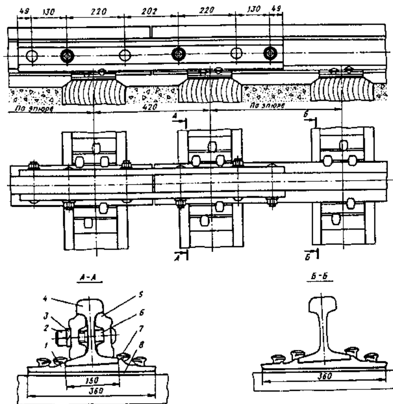
Рис. 3.1. Стыковое и промежуточное костыльное скрепление при рельсах Р65, Р75: 1 — подкладка Д65; 2 — гайка М27; 3 — пружинная одновитковая шайба; 4 — рельс типа Р65; 5 — двухголовая накладка; 6 — путевой болт М27×160; 7 — путевой костыль; 8 — прокладка под подкладку
