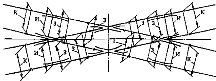
Рис. 3.11. Места контрольных измерений ширины колес в прямолинейных косоугольных глухих пересечениях
