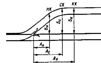
Рис. П.4.1. Схема разбивки закрестовинной кривой
