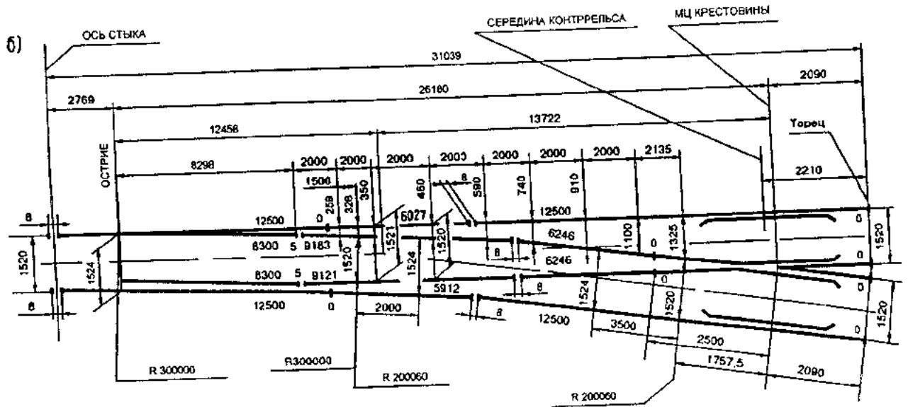
Рис. 5.14. Эпюра укладки (а) и схема разбивки (б) стрелочного перевода типа Р65 марки 1/9 на железобетонных брусках. Проекты 2769 и 2215
