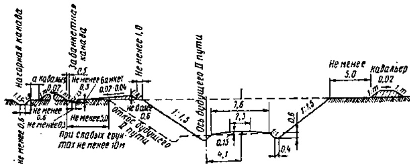
Рис. П.6.2. Выемка глубиной до 12 м с шириной основной площадки 7,6 м при поперечном уклоне местности не круче 1:3
