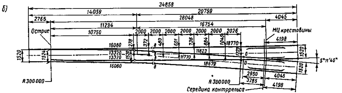
Рис. 5.10. Эпюры укладки (правосторонняя и левосторонняя) (а) и схема разбивки (б) стрелочного перевода типа Р65 марки 1/11 на железобетонных брусьях. Проект 2750
