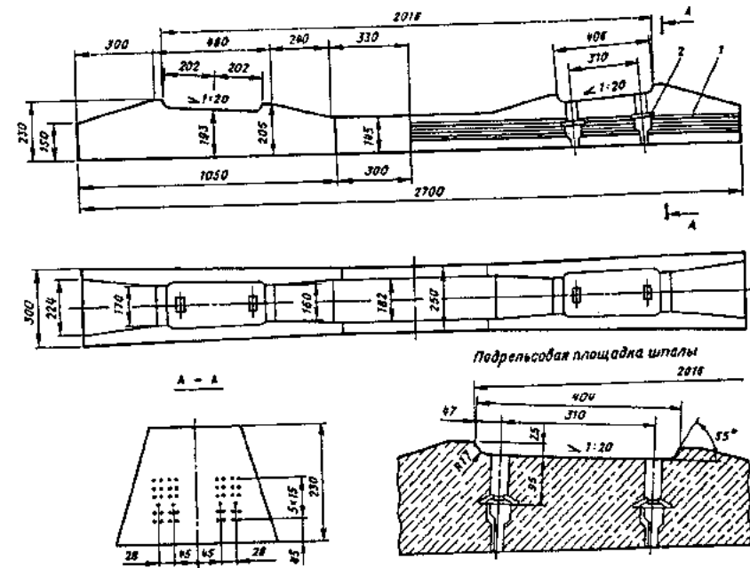
Рис. П.3.3. Железобетонная шпала типа ШП-1: 1 — арматура; 2 — закладная шайба
