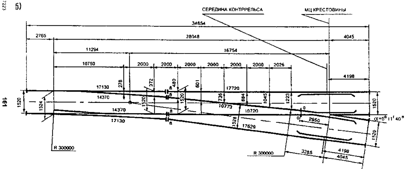
Рис. 5.6. Эюра укладки (а) и схема разбивки (б) стрелочного перевода типа Р65 марки 1/11. Проекты 2717 и 2718
