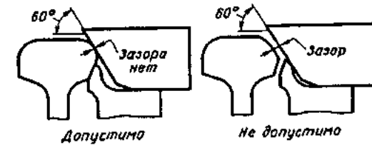
Рис. 3.22. Проверка шаблоном КОР взаимного положения остяжков и рамных рельсов
