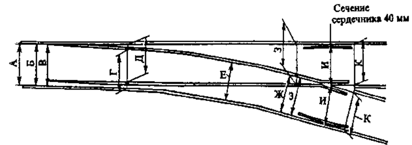
Рис. 3.8. Места контрольных измерений ширины колес на обыкновенных стрелочных переводах
