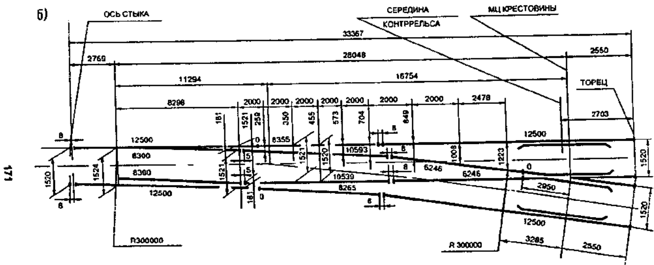
Рис. 5.11. Эпюра укладки (а) и схема разбивки (б) стрелочного перевода типа Р65 марки 1/11 на железобетонных брусках. Проекты 2768 и 1740
