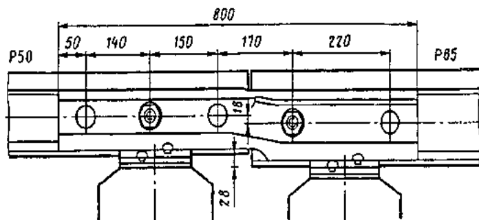
Рис. 3.4. Переходной стык Р65/Р50
