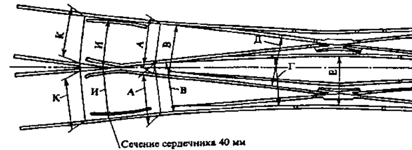
Рис. 3.9. Места контрольных измерений ширины колес на двойных перекрестных стрелочных переводах
