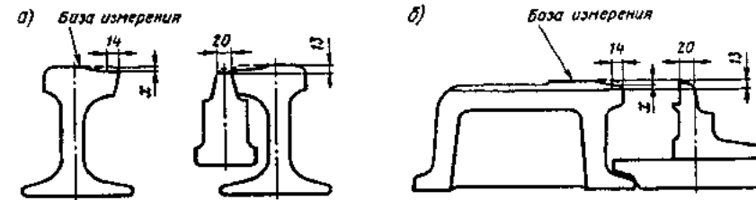
Рис. 3.21. Измерение вертикального износа x усювиков острой (а) и тупой (б) крестовины с подвижным (поворотным) сердечником
