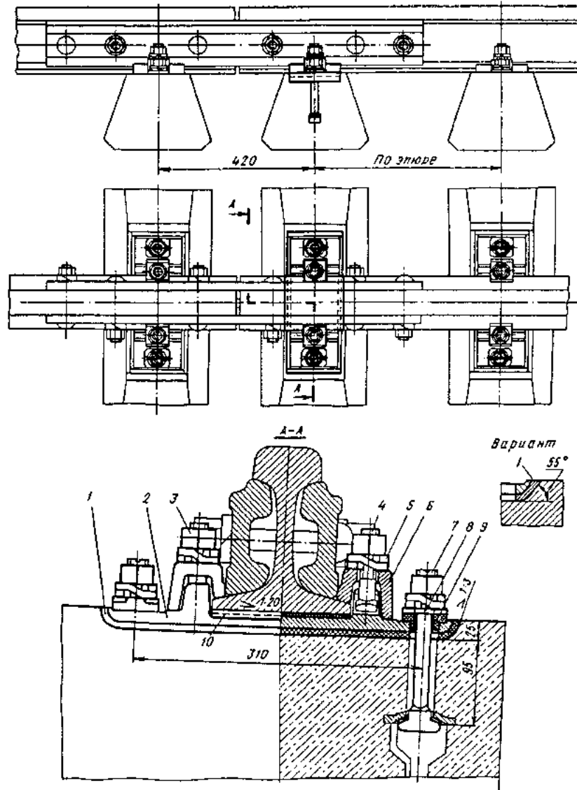
Рис. 3.2. Стыковое и промежуточное скрепление КБ65 на железобетонных шпалах с рельсами Р65 и Р75:
