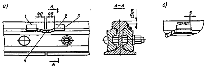
Рис. 3.34. Схема установки (а) и приварки (б) медного соединителя фартучного типа к головке рельса: 1 — шов, выполняемый ручной электродуговой сваркой; 2 — фартук; 3 — наконечник (манжета); 4 — гибкий трос МГГ-70
