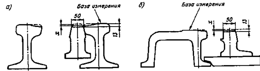
Рис. 3.20. Измерение вертикального износа x сердечника острой (а) и тупой (б) крестовины с подвижным сердечником
