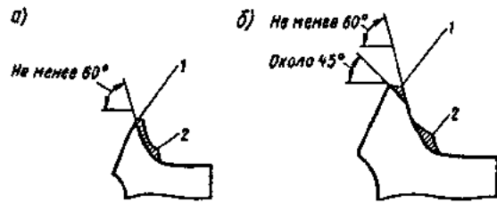
Рис. 3.24. Профиль зачистки выкошенного остряка: а — до первой тяги; б — за первой тягой на участке до сечения остряка 20 мм; 1 — выкрашивание головки; 2 — горизонтальный уступ
