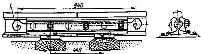
Рис. 3.36. Рельсовый стык со штепсельным соединителем (1)
