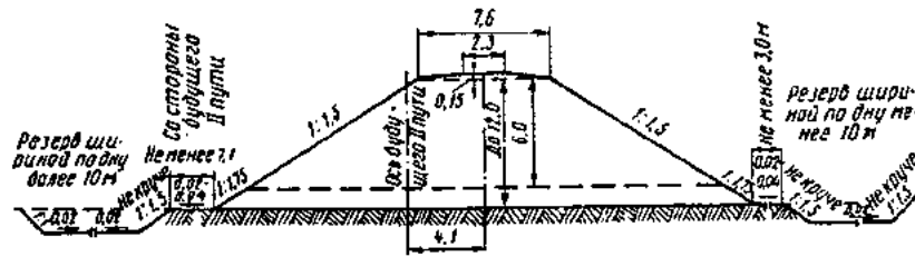
Рис. П.6.1. Насыпь высотой до 12 м с шириной основной площадки 7,6 м при поперечном уклоне местности не круче 1:5
