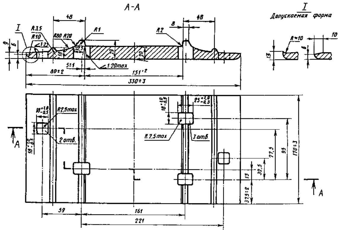
Рис. П.2.7. Подкладка стрелочная СД-65 костьельного скрепления
