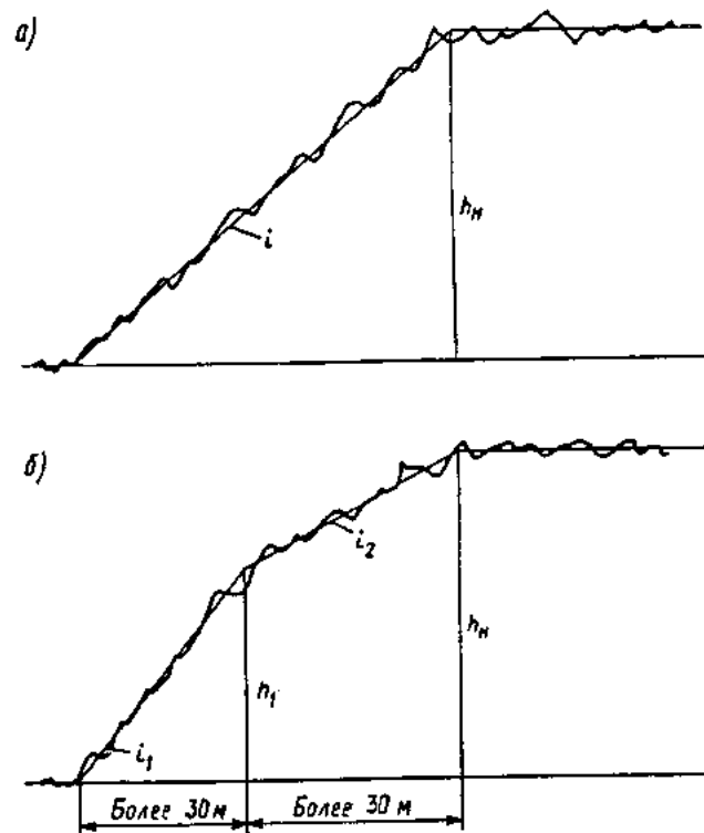
Рис. 2.1. Отводы возвышения наружного рельса кривой на ленте путеизмерителя: а — номинальный отвод ( i ); б — допустимый отвод ( i_1, i_2 ) в процессе текущего содержания ( V = 120 \text{ км/ч} )
