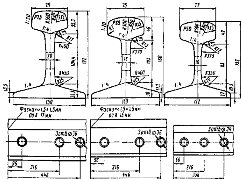
Рис. П.1.1. Рельсы типа P75, P65, P50
